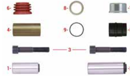
Kısa Pim 34x80 Uzun Pim 36x113,70
